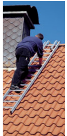
Firstüberwurfbügel mit Leiter montiert
