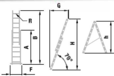
Mehrzweckleiter
